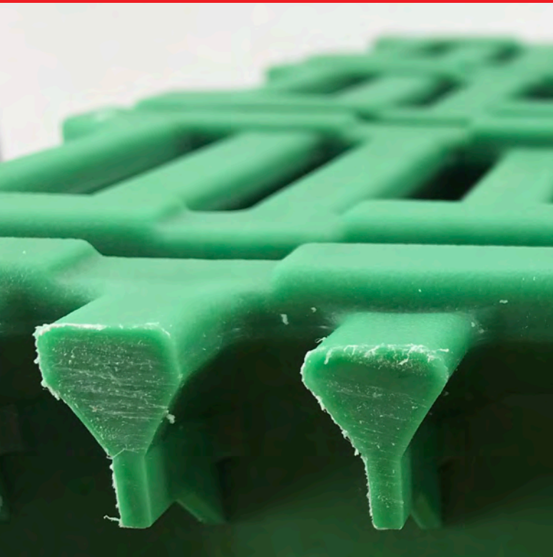
Sección transversal: sin residuos durante la limpieza gracias a su forma cónica
