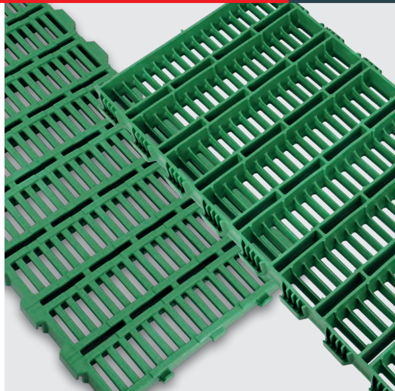
Rejilla para cerdas WEDA 800 x 400 mm; hasta peso máx. de animal de 350 kg
