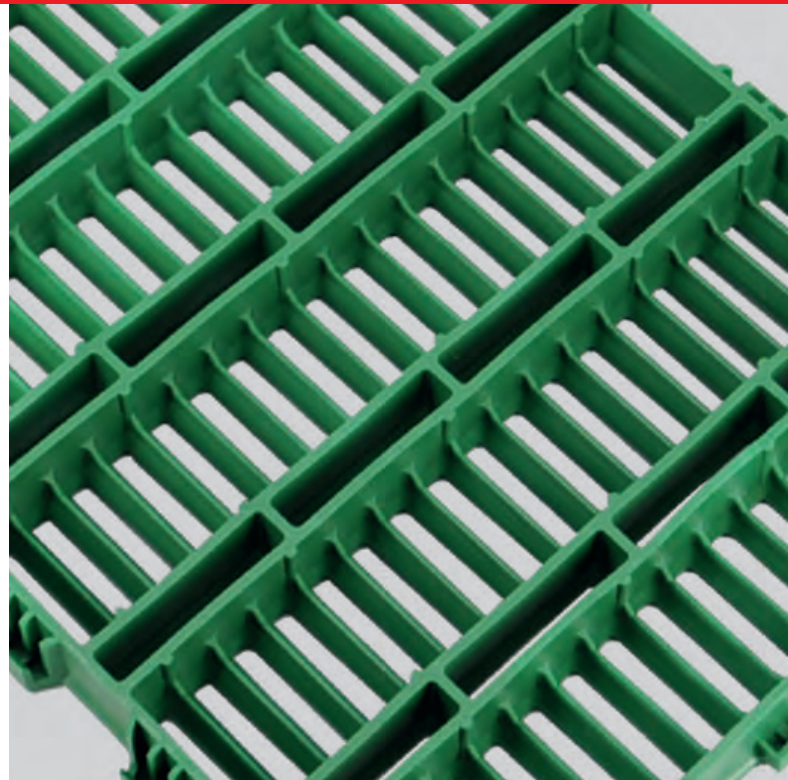
Las pasarelas dobles permiten realizar cortes individuales en caso necesario
